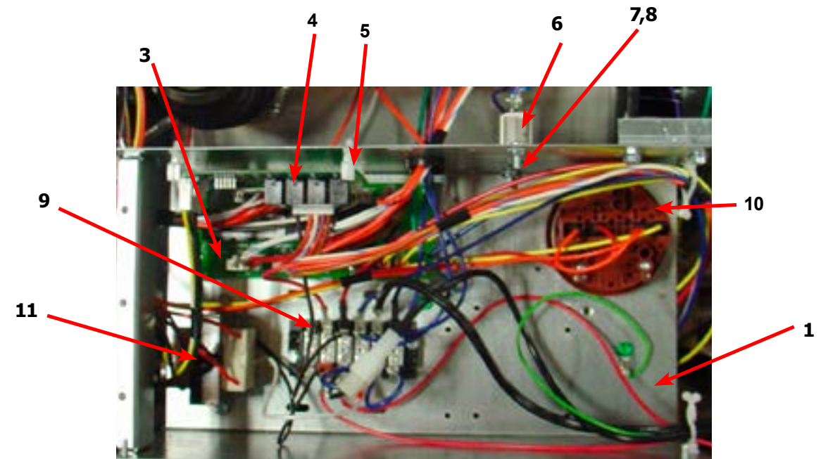
120 Volt Trough W/O step down Transformer
