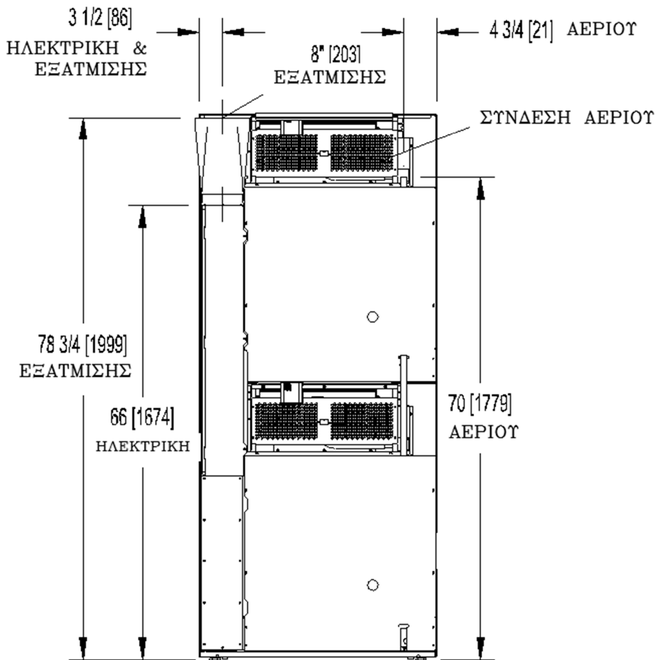
Εικόνα 6-6 Πίσω όψη T-50X2
