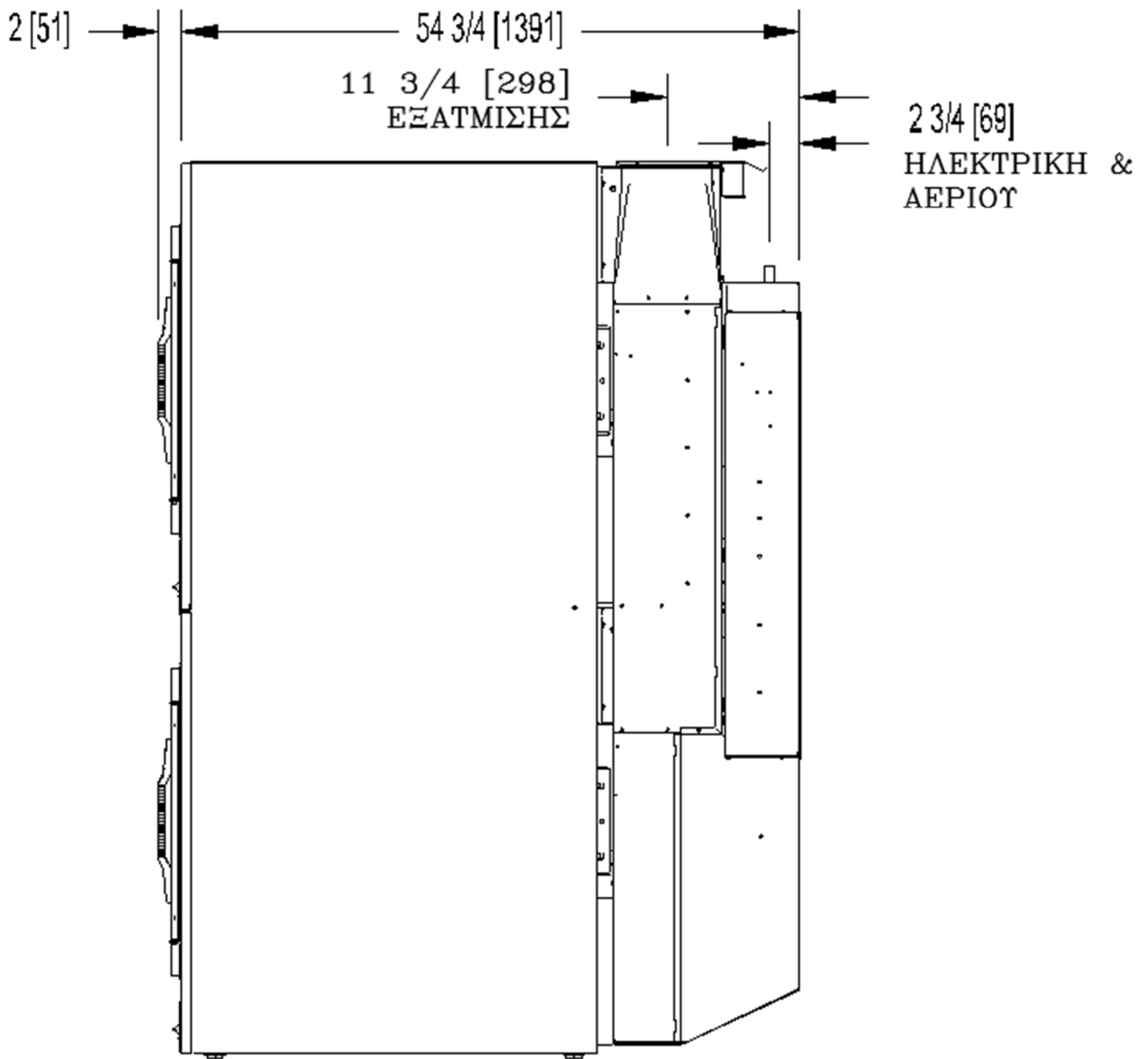
Εικόνα 6-5 Πλευρική όψη T-50X2
