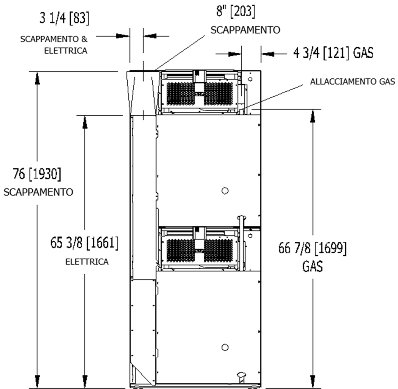
Figura 6-3 Vista posteriore T-30X2
