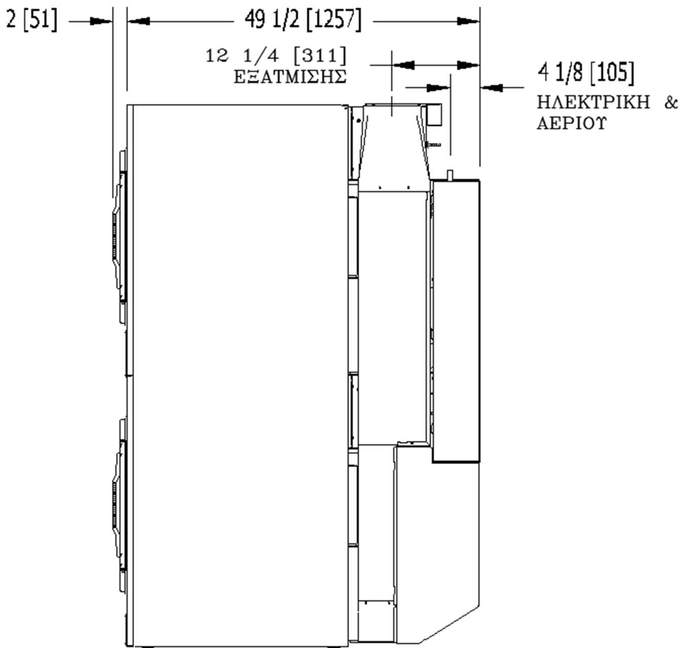
Εικόνα 6-2 Πλευρική όψη T-30X2
