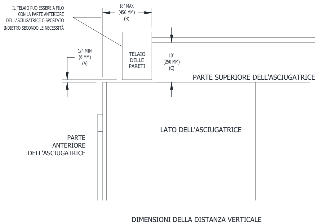
Figura 7-1 Dimensioni della distanza verticale
