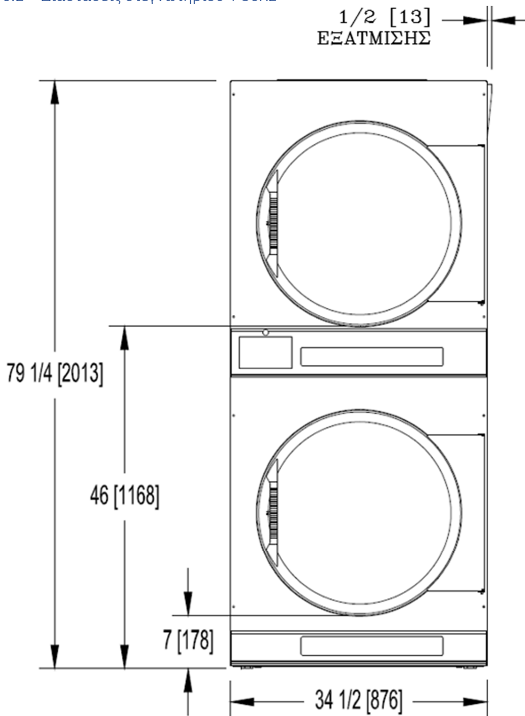
Εικόνα 6-4 Μπροστινή όψη T-50X2
