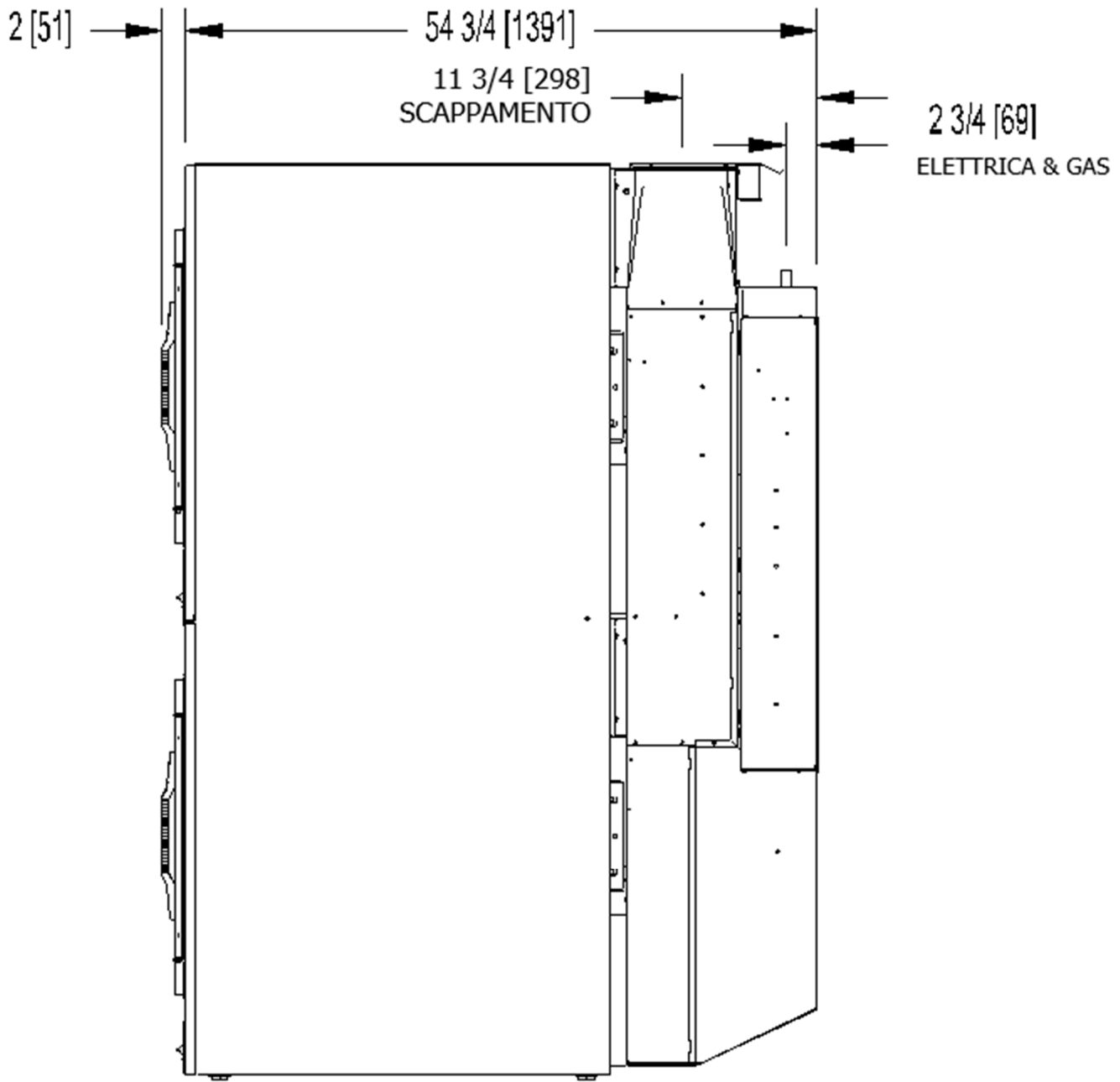
Figura 6-5 Vista laterale T-50X2
