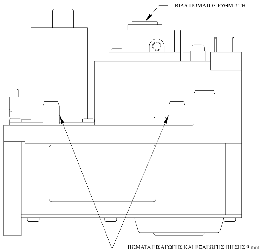
Εικόνα 7-3 Προσαρμογή ρυθμιστή πίεσης
