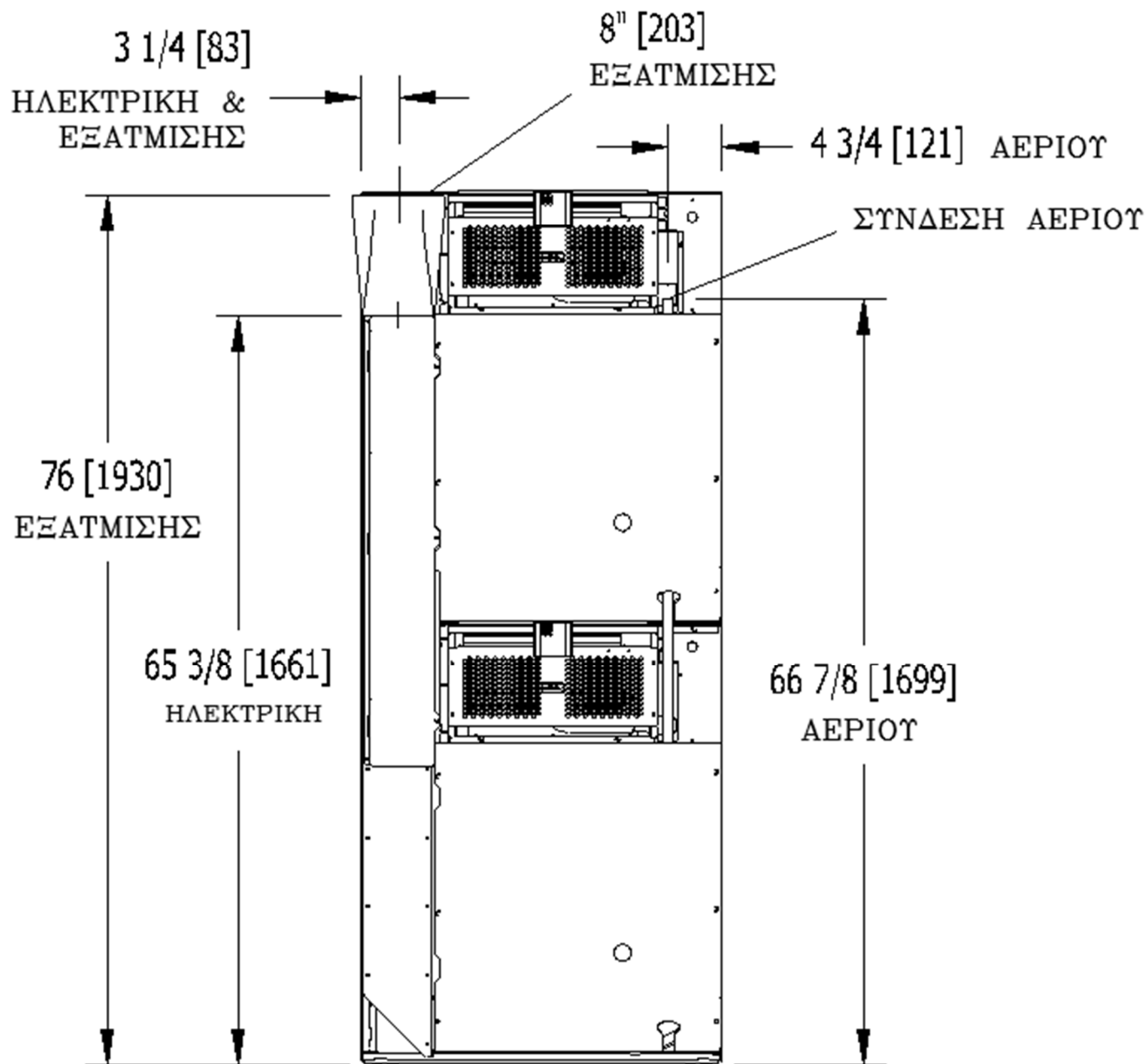
Εικόνα 6-3 Πίσω όψη T-30X2
