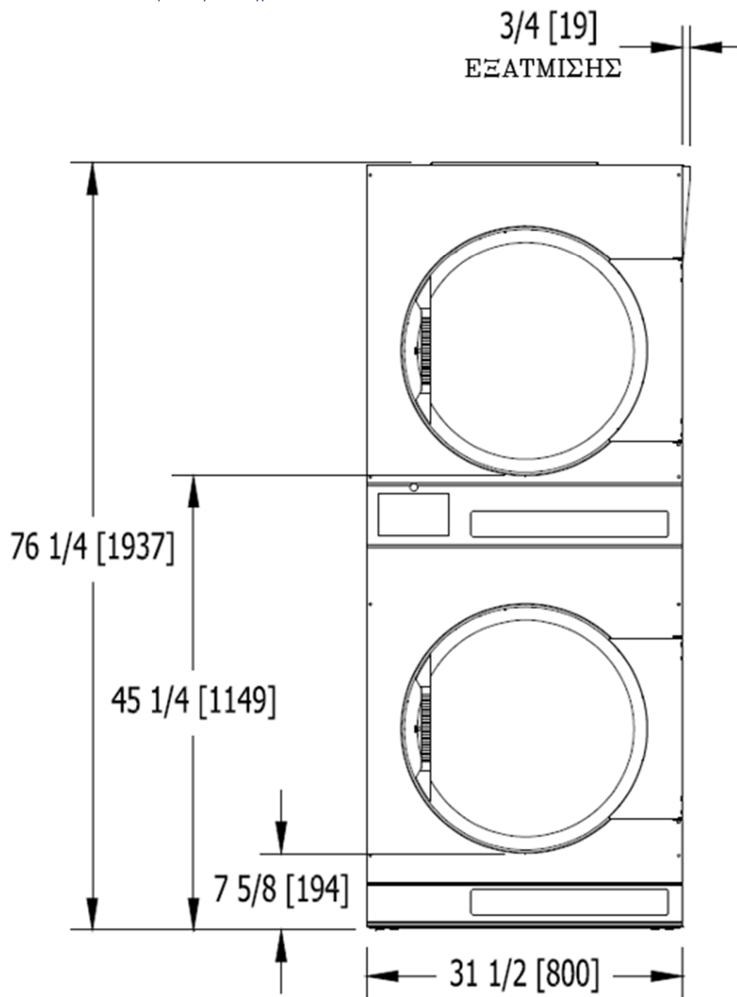
Εικόνα 6-1 Μπροστινή όψη T-30X2
