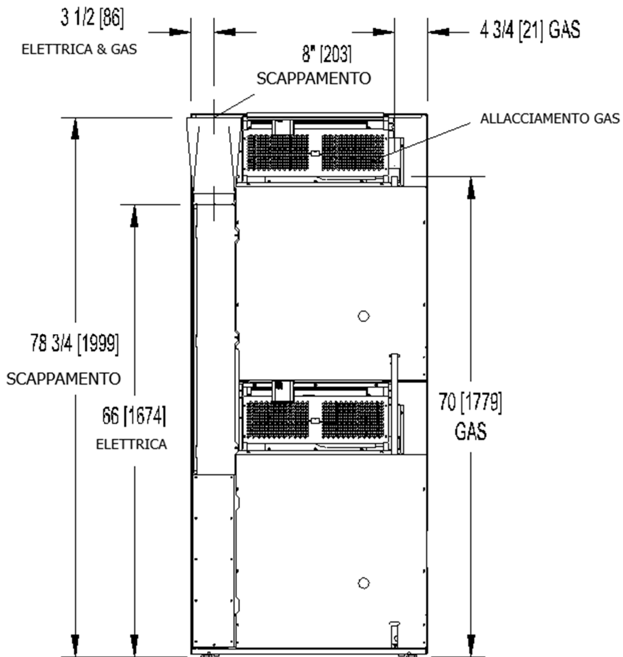
Figura 6-6 Vista posteriore T-50X2
