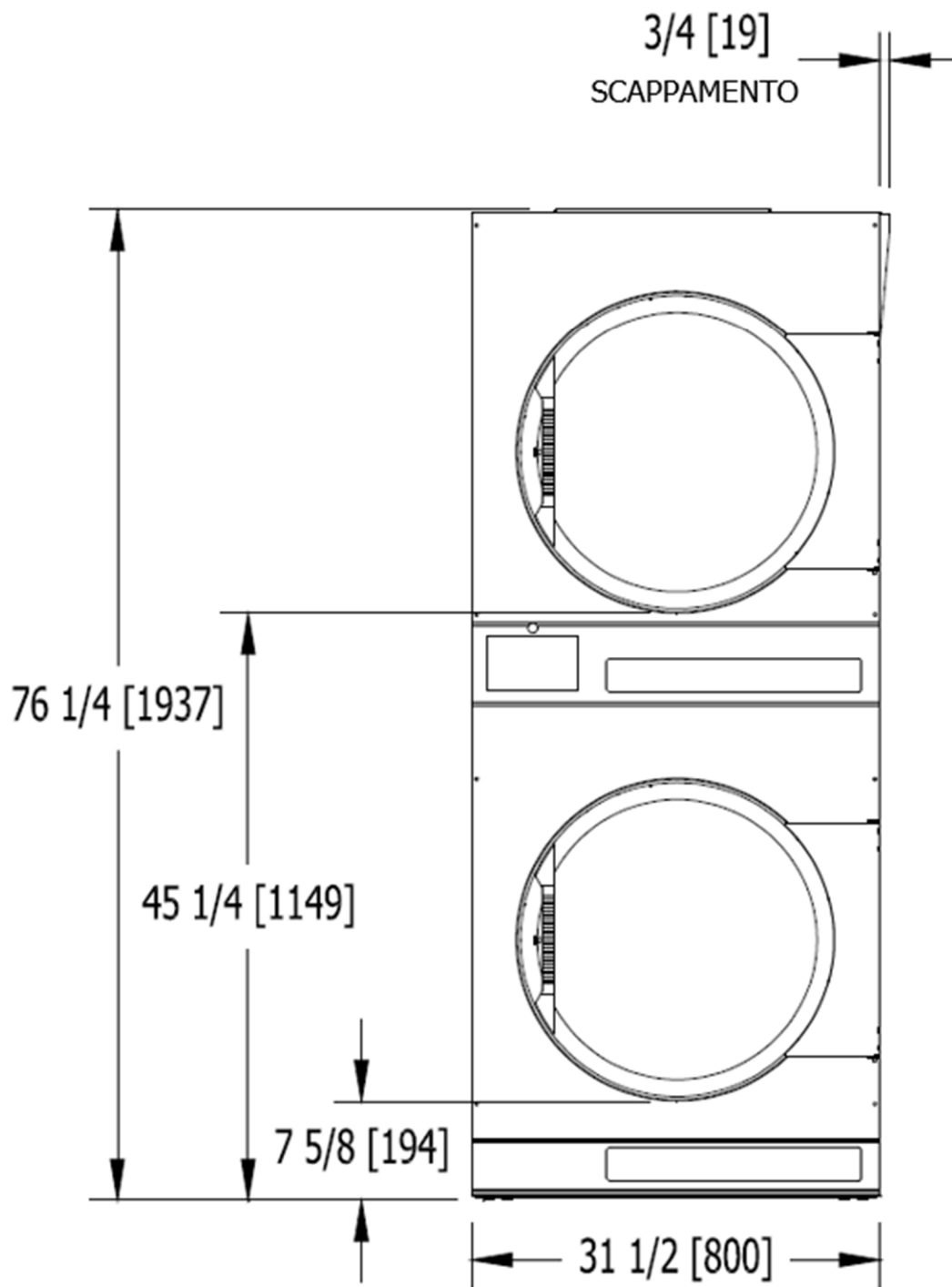
Figura 6-1 Vista frontale T-30X2
