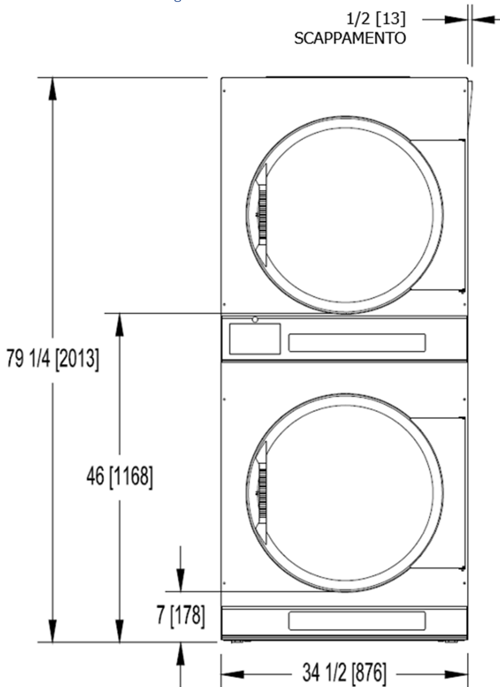
Figura 6-4 Vista frontale T-50X2
