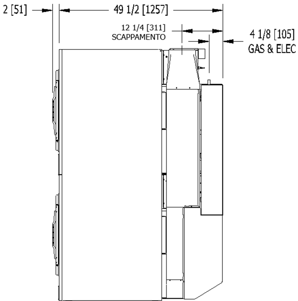
Figura 6-2 Vista laterale T-30X2
