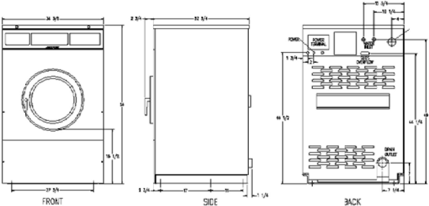
T-750 Machine Dimensions
