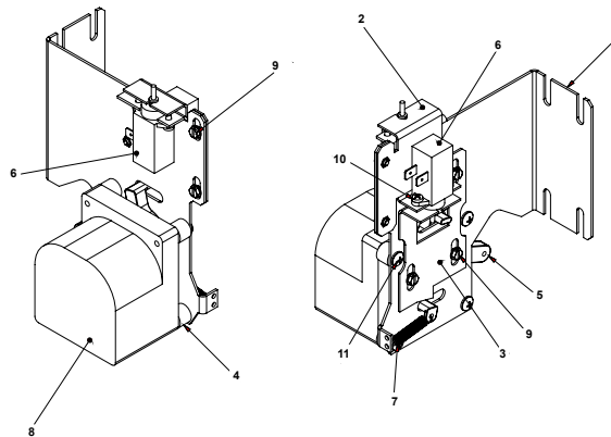
Door Lock Gear Motor
