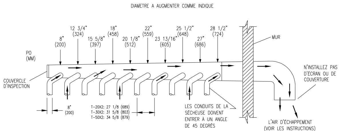
FIGURE 3- Sècheur Épaisant à l'aide d'un conduit d'évacuation principal
